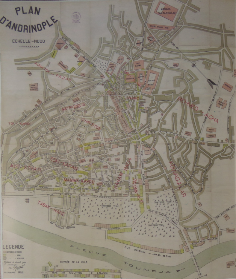
PLAN D'ANDRINOPLE-EDİRNE ŞEHİR PLANI 205x100 cm, 1/1000 ölçek, renkli orijinal çizim, Aralık 1905 tarihli ipek kağıda orijinal çizim şehir planı. Edirne Valiliği Arşivi
